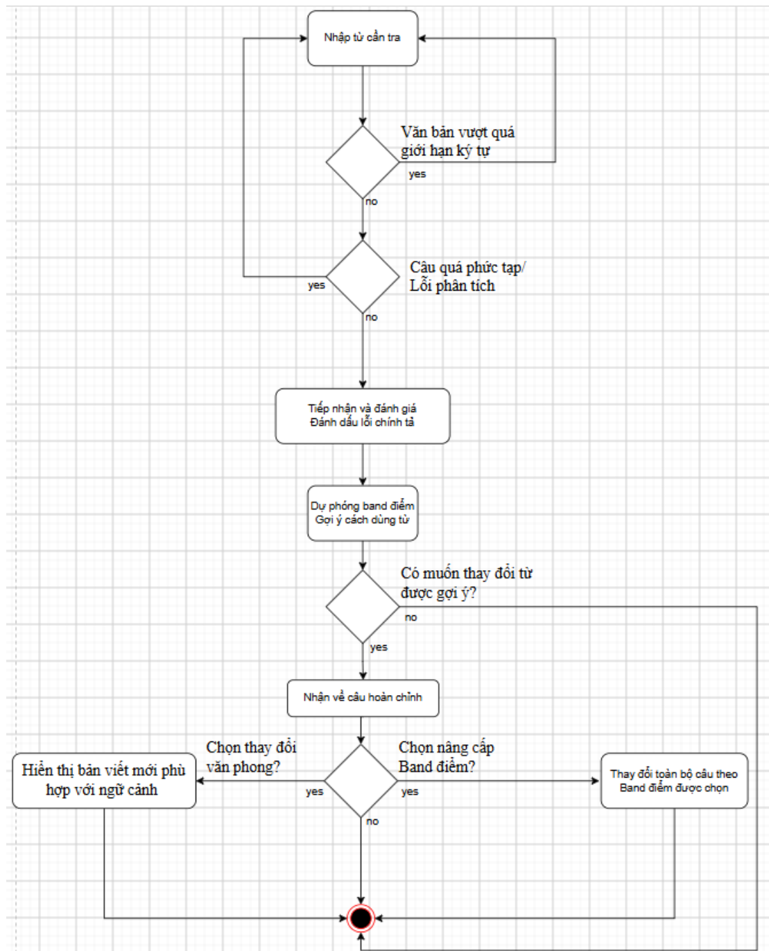
Hình 3 Activity Diagram UC3
