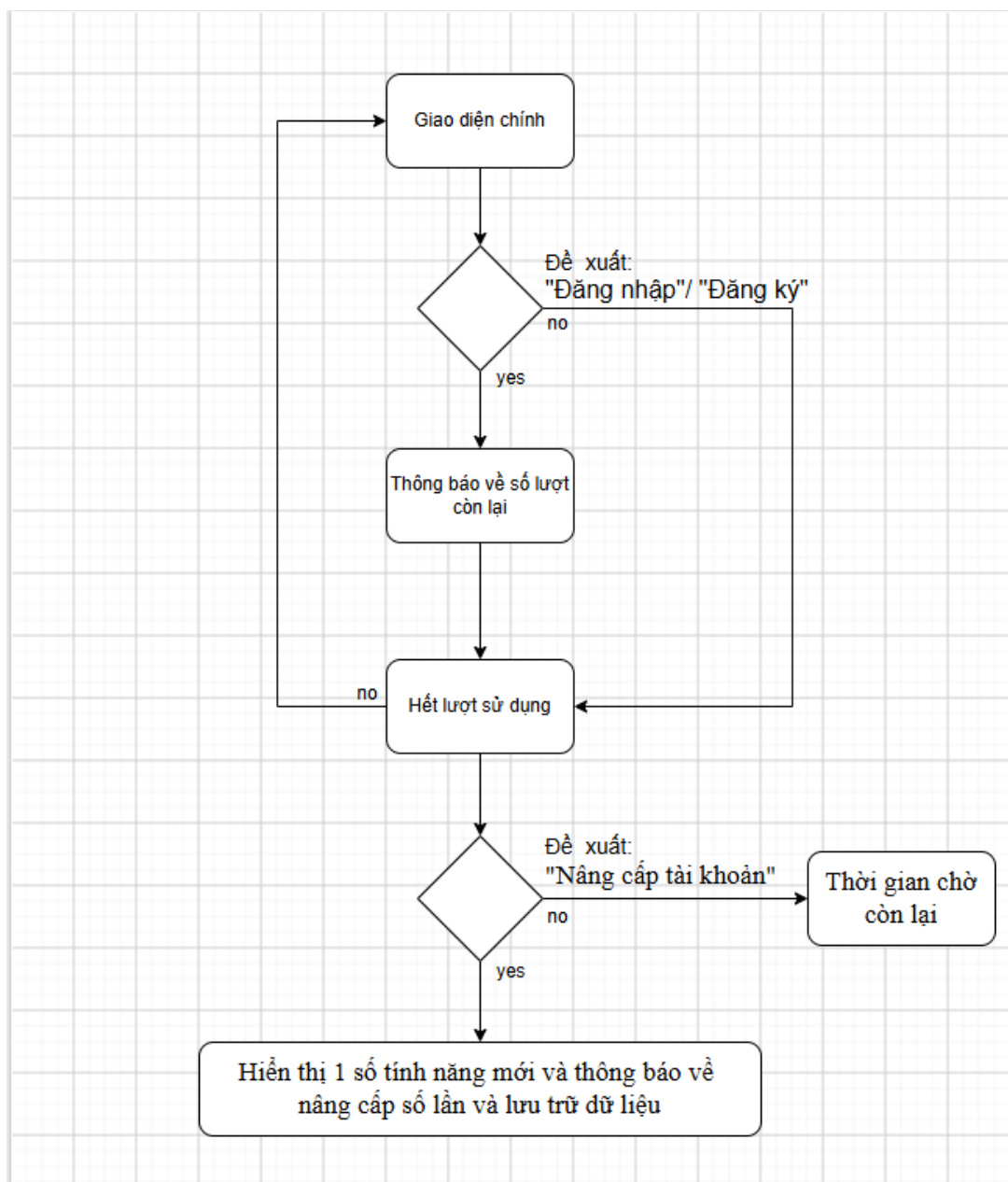
Hình 1 Activity Diagram UC1
