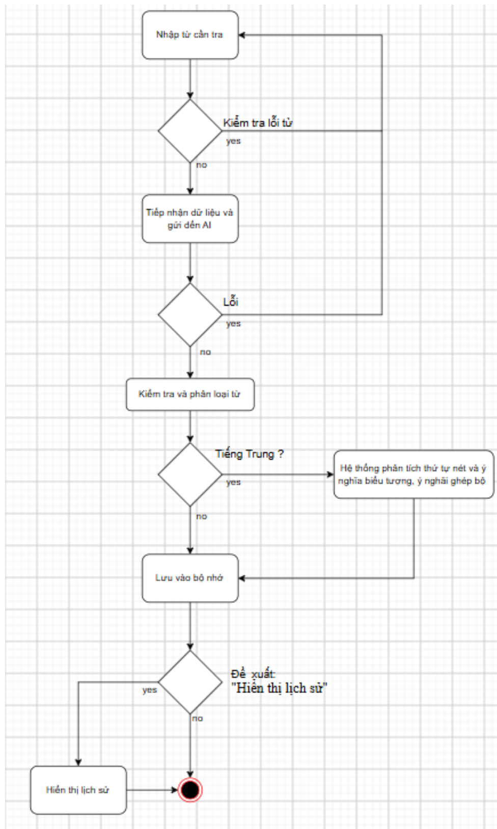
Hình 2 Activity Diagram UC2
